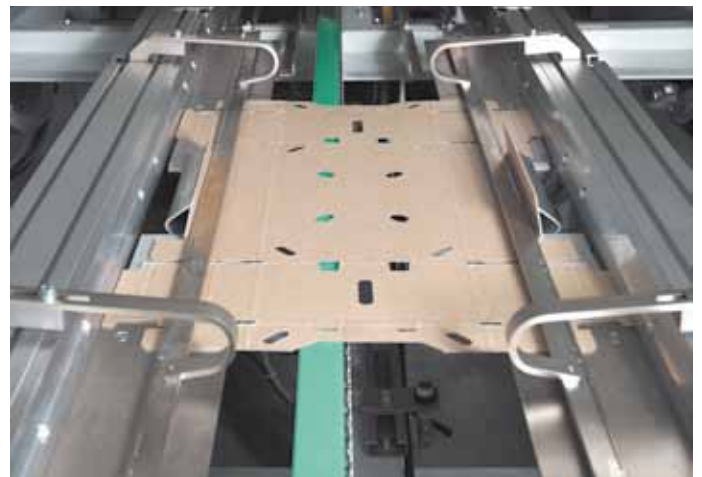
Prebending system Gruppo pre-sneratura Vorbiegeeinheit Grupo pre-deformación
