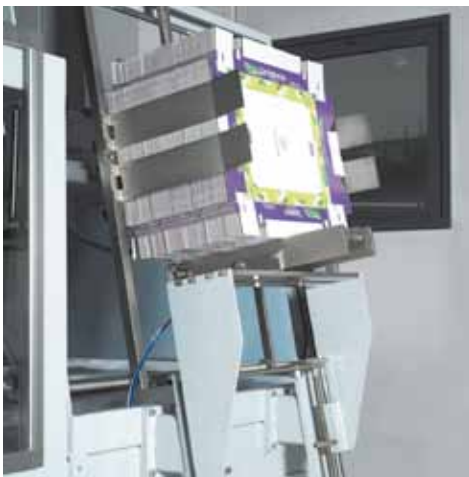
Vertical side infeed system Gruppo magazzino laterale Seitliche Magazineinheit Grupo almacén lateral
