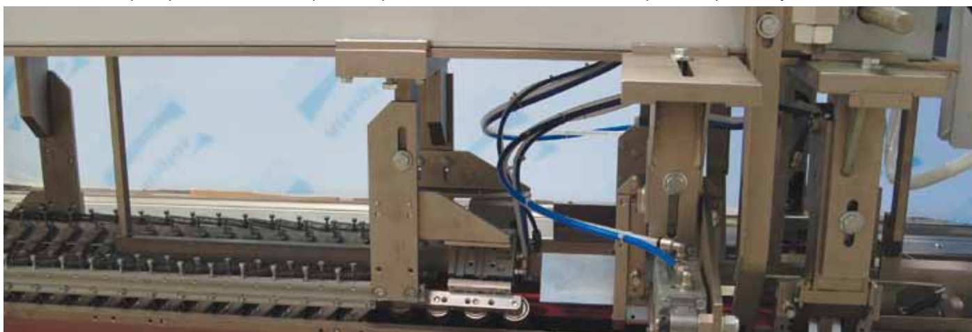
Long and short side doubling Raddoppi testate e fiancate Verdoppelte Kopfseiten und Seitenwände Paredes dobles en partes superiores y en laterales
