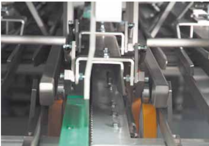
Wheels conveyor Ruote avanzamento Vorlaufräder Ruedas de avance
